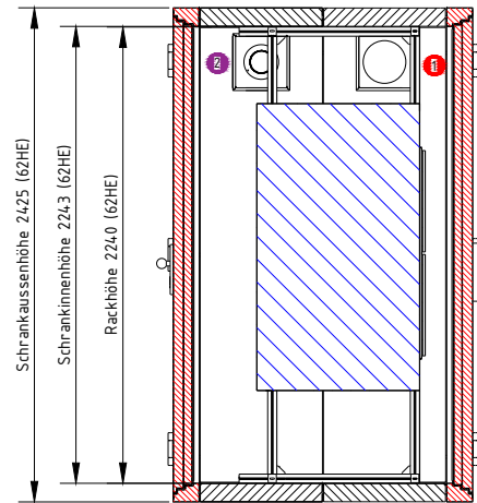
B-B ( 1 : 25 )
