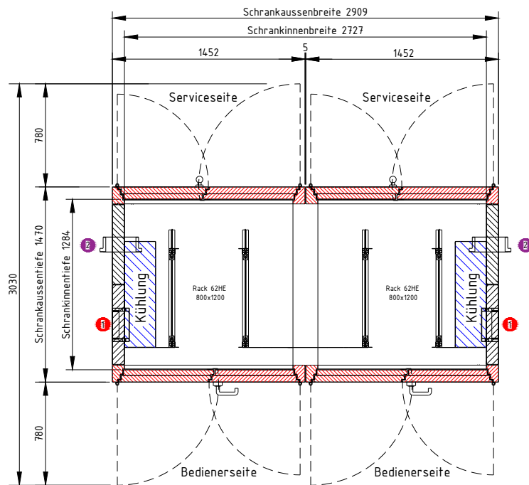
A-A ( 1 : 25 )
