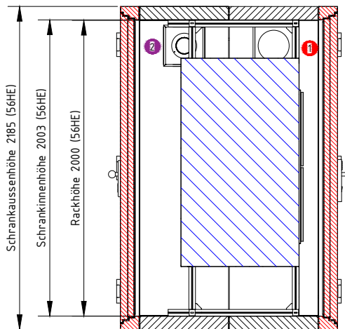
B-B ( 1 : 25 )
