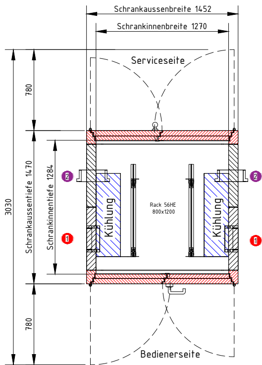
A-A ( 1 : 25 )
