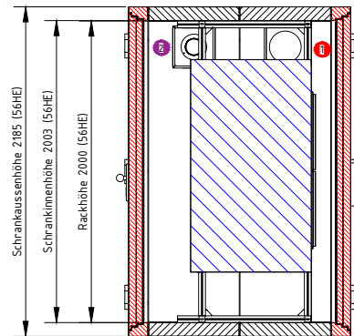
B-B ( 1 : 25 )
